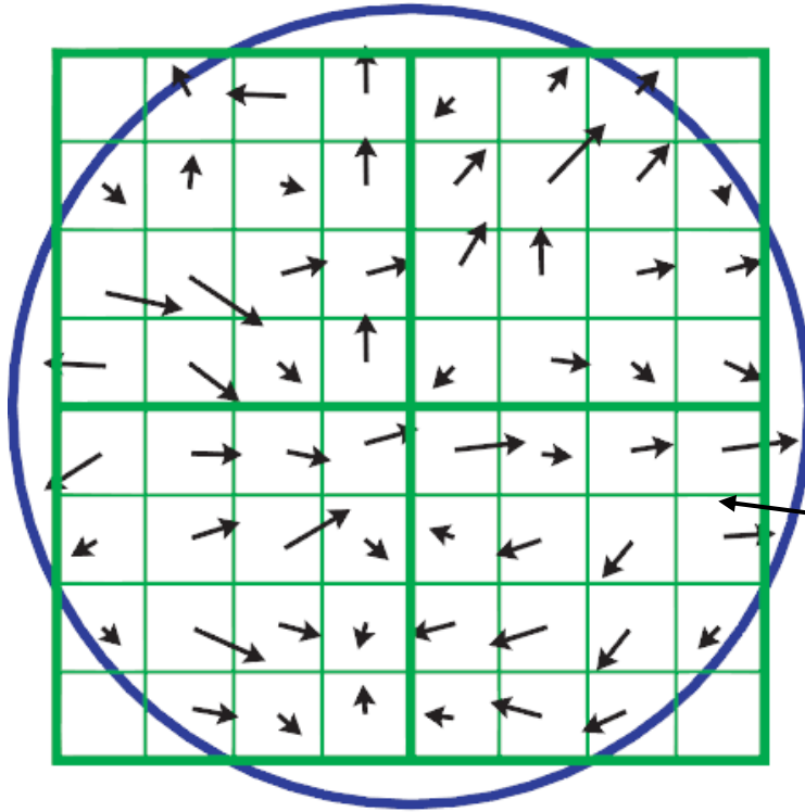
Image gradients
