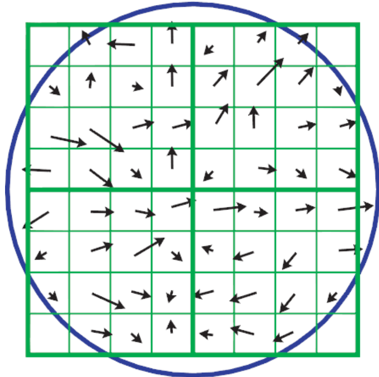
Image gradients
